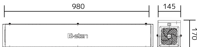
外形寸法 (mm)
